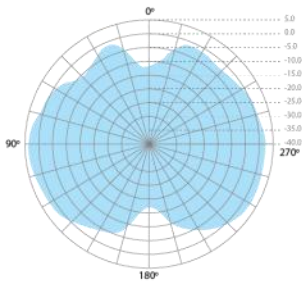
2.4GHz 2D 無線場形 @ 垂直方向
