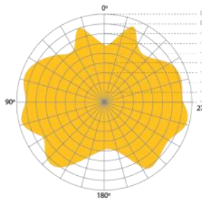
5GHz 2D 無線場形 @ 垂直方向
