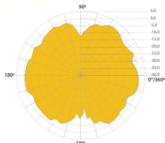
5GHz 2D 無線場形 @ 垂直方向
