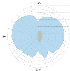
2.4GHz 2D 無線場形 @ 垂直方向
