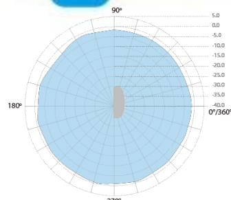
2.4GHz 2D 無線場形 @ 水平方向
