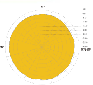
5GHz 2D 無線場形 @ 水平方向
